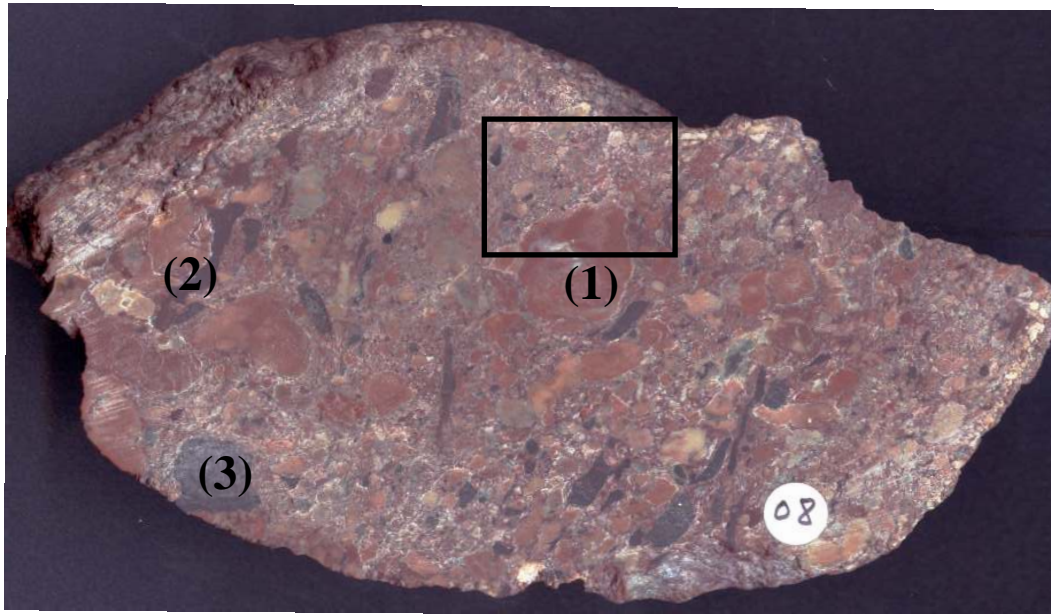
07_1 : Conglomérat à matrice argilo ferrugineuse échelle 1/1
